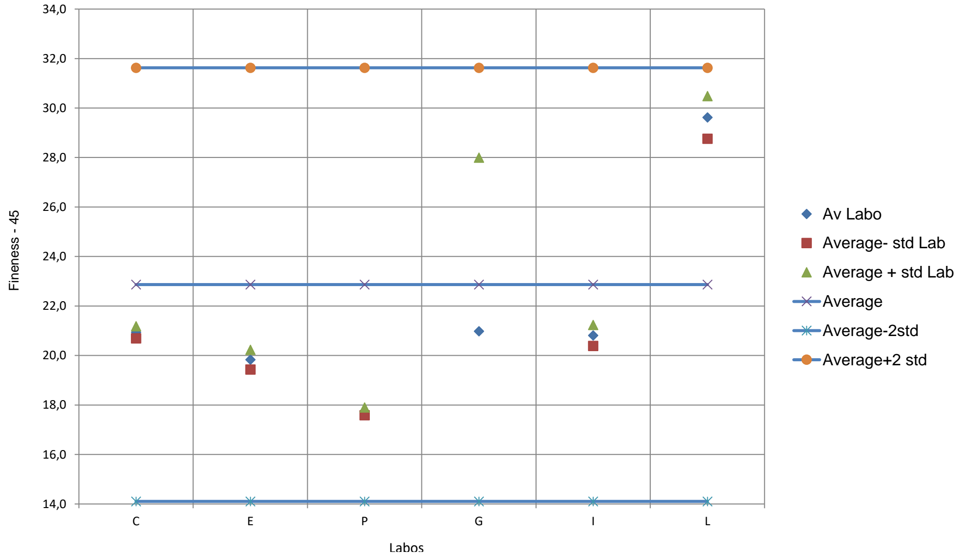
BE-CERT Round Robin Test Fly-Ash - 2015-2017 - Fineness
