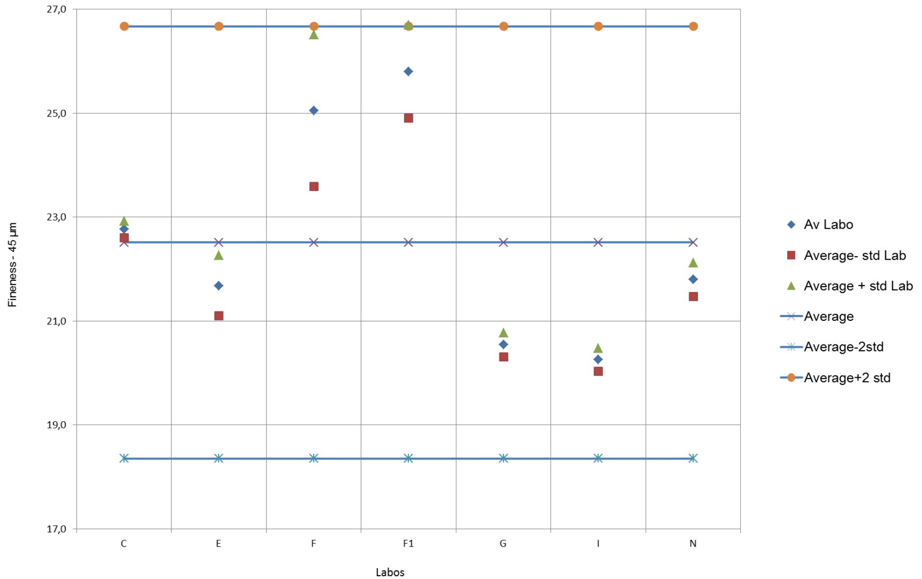
BE-CERT Round Robin Test Fly-Ash - 2013-2015 - Fineness
